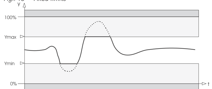
Fig.: 18 Fixed limits
