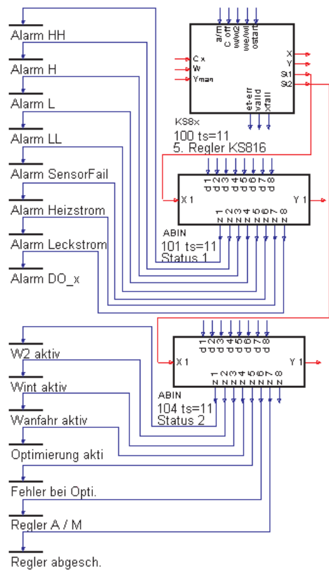
Beispielengineering zur Auswertung St1/ St2
